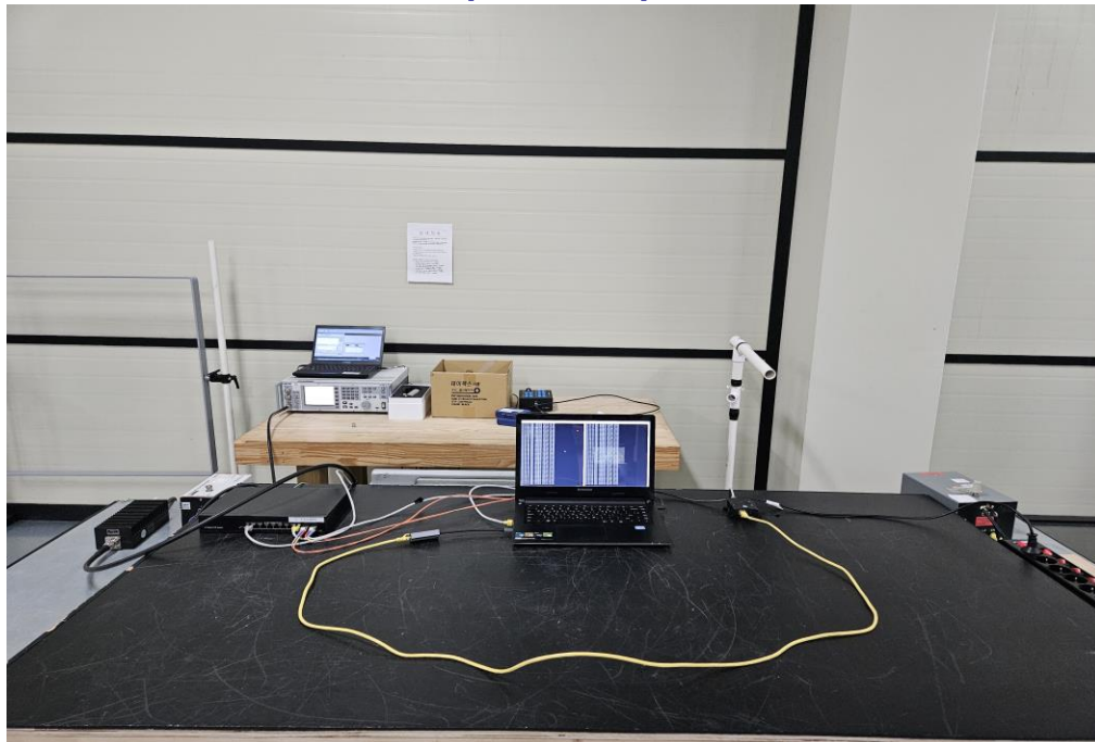
[ 데이터 포트 ]
