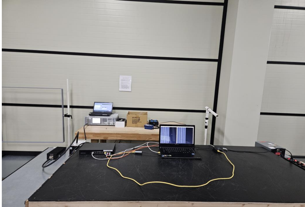
[ 전원 포트 ]
